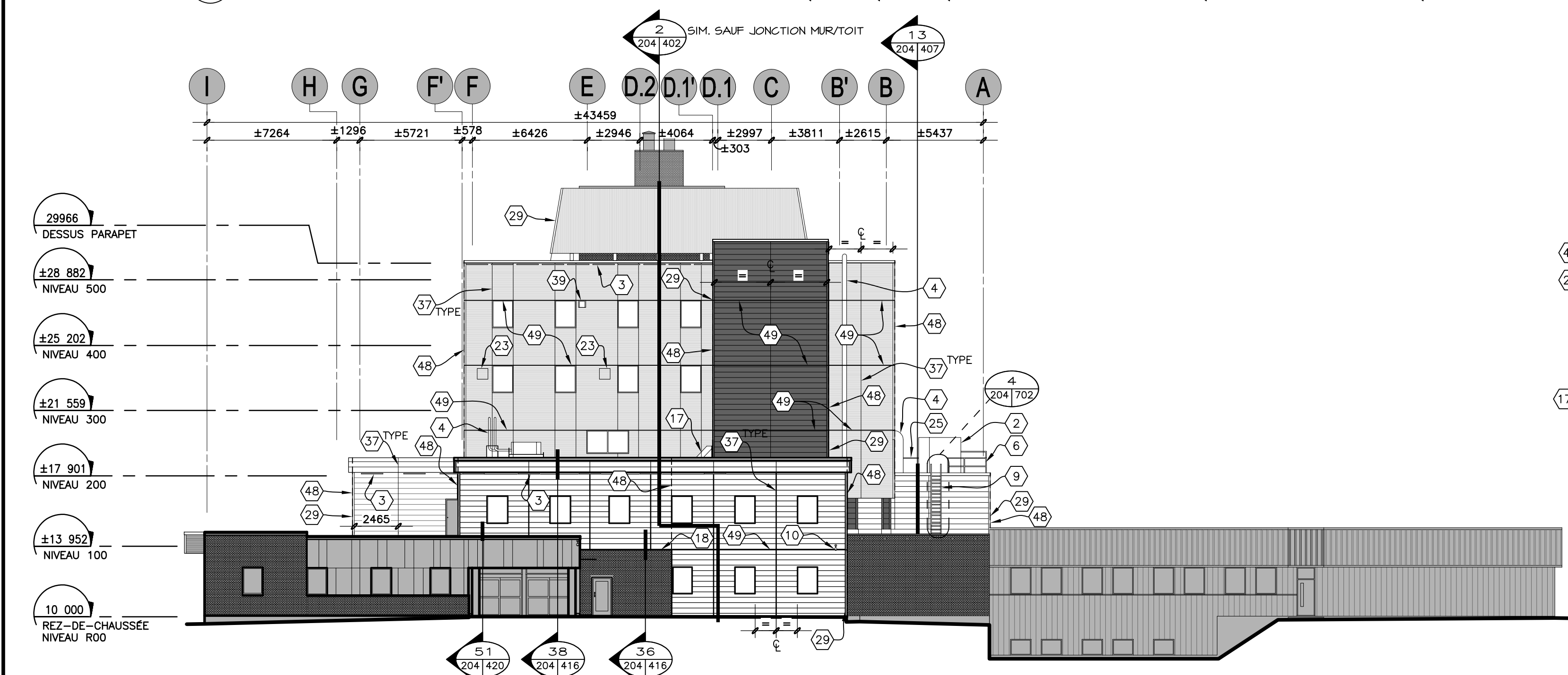
G ÉLEVATION EST - CONSTRUCTION 1:200mm
