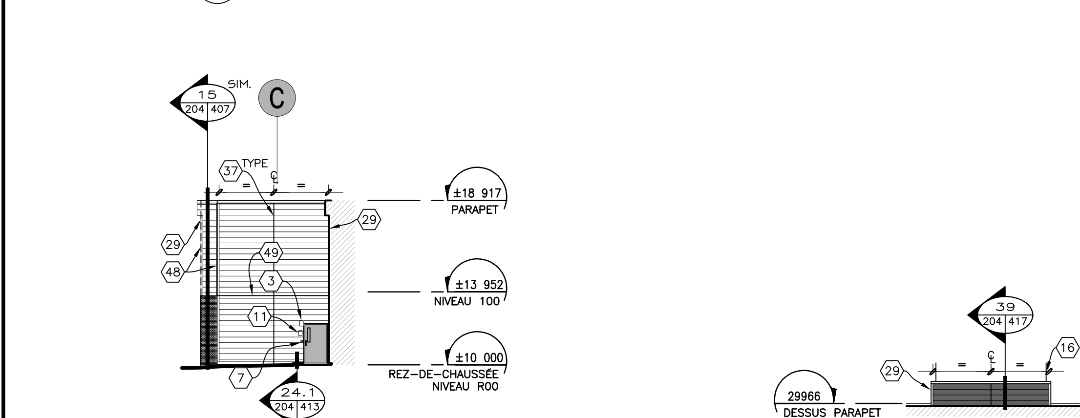
I ÉLEVATION OUEST PARTIELLE - CONSTRUCTION 1:200mm
