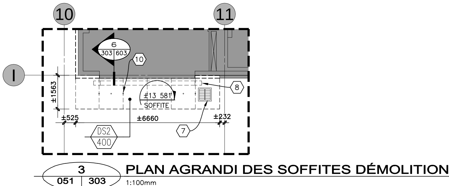
PLAN AGRANDI DES SOFFITES DÉMOLITION
