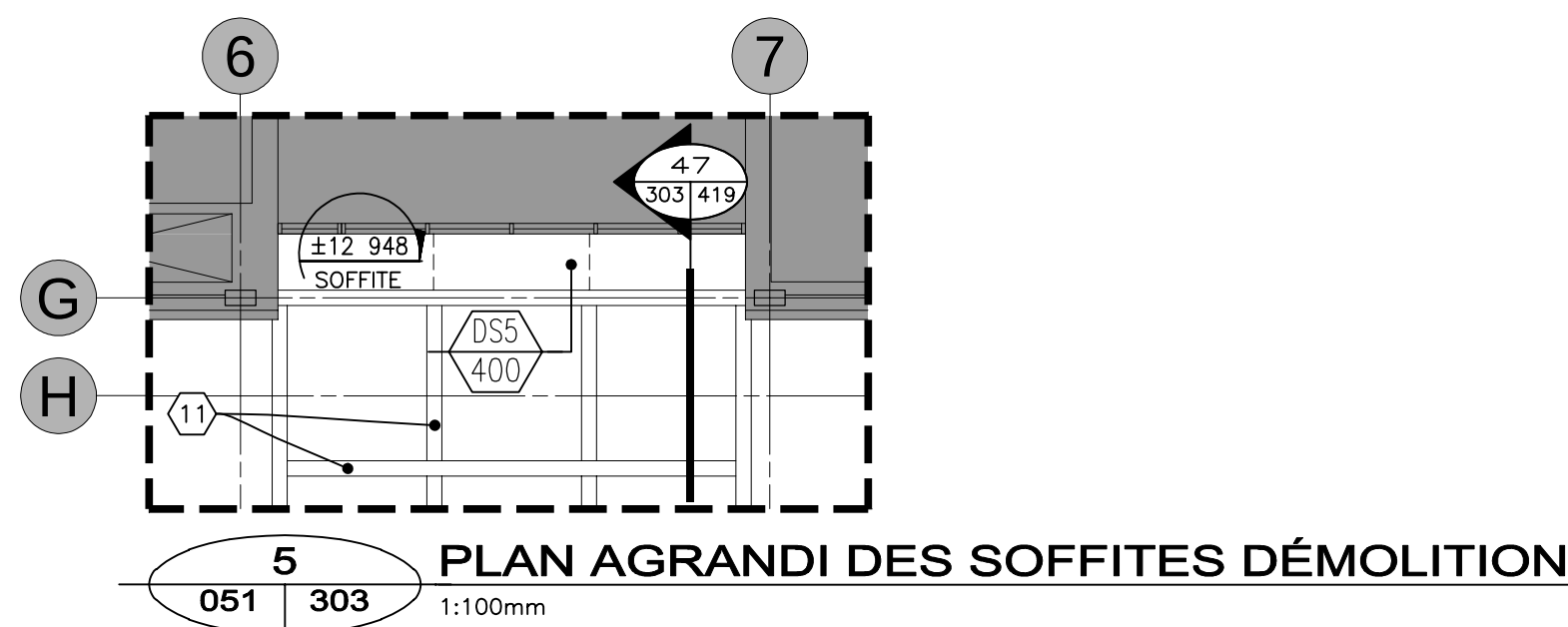
PLAN AGRANDI DES SOFFITES DÉMOLITION
